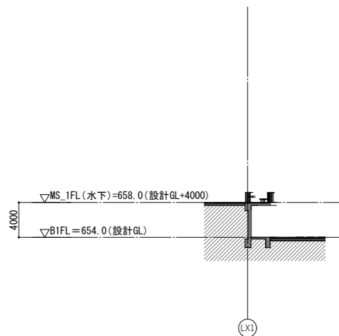
北サイドスタンド K-K断面図 (LY7-8)
