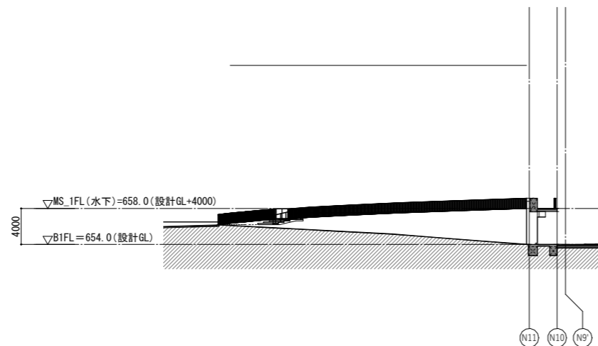
北サイドスタンド L-L断面図 (LY13-14)
