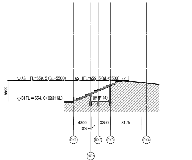
南サイドスタンド H-H断面図 (RY10-11)
