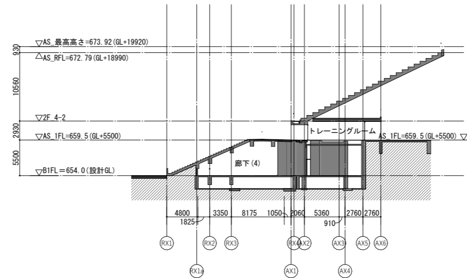
南サイドスタンド I-I断面図 (AY6)
