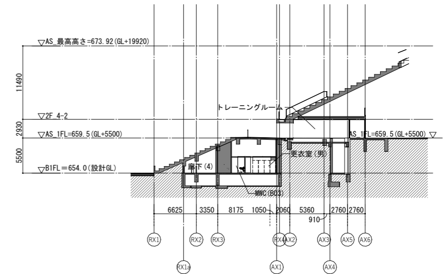
南サイドスタンド J-J断面図 (AY6-7)
