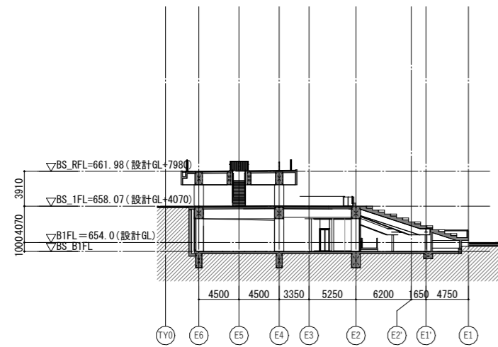
D-D断面図 (N5-6)
