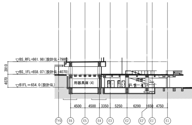
E-E断面図 (N6-7)
