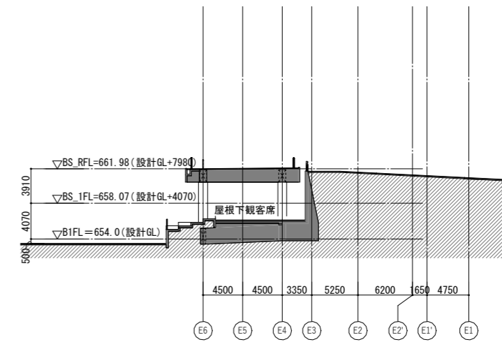
F-F断面図 (N10'-13)
