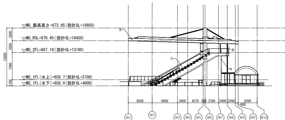
北立面図
