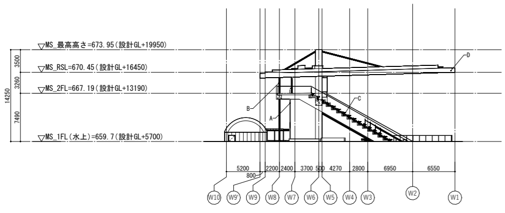
南立面図
